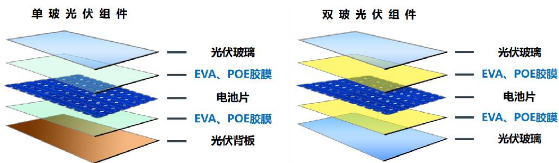
图：单/双玻组件结构示意图
